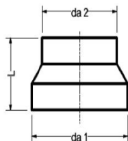
تبدیل هم مرکز پلی اتیلن مطابق استاندارد ۱۴۴۲۷/ISIRI/PE۱۰۰
