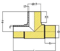
سه راهی پلی اتیلن مطابق استاندارد PE100/ISIRI14427
