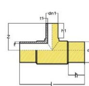
سه راهی پلی اتیلن مطابق استاندارد PE100/ISIRI14427
